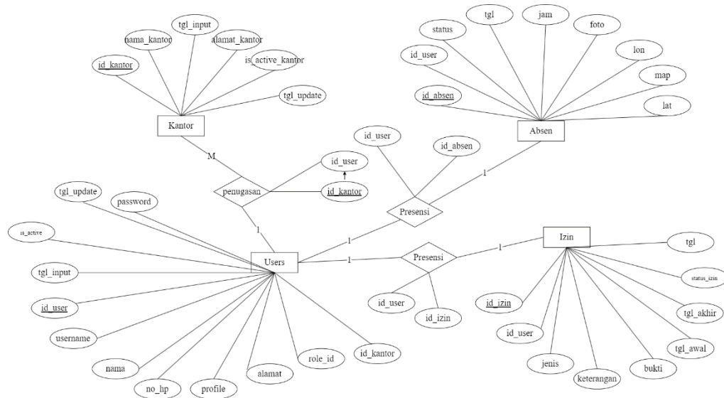
Gambar 3. Rancangan ERD
